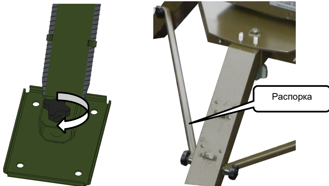
Рисунок 21 – Установка подпятников на опорные лапы
