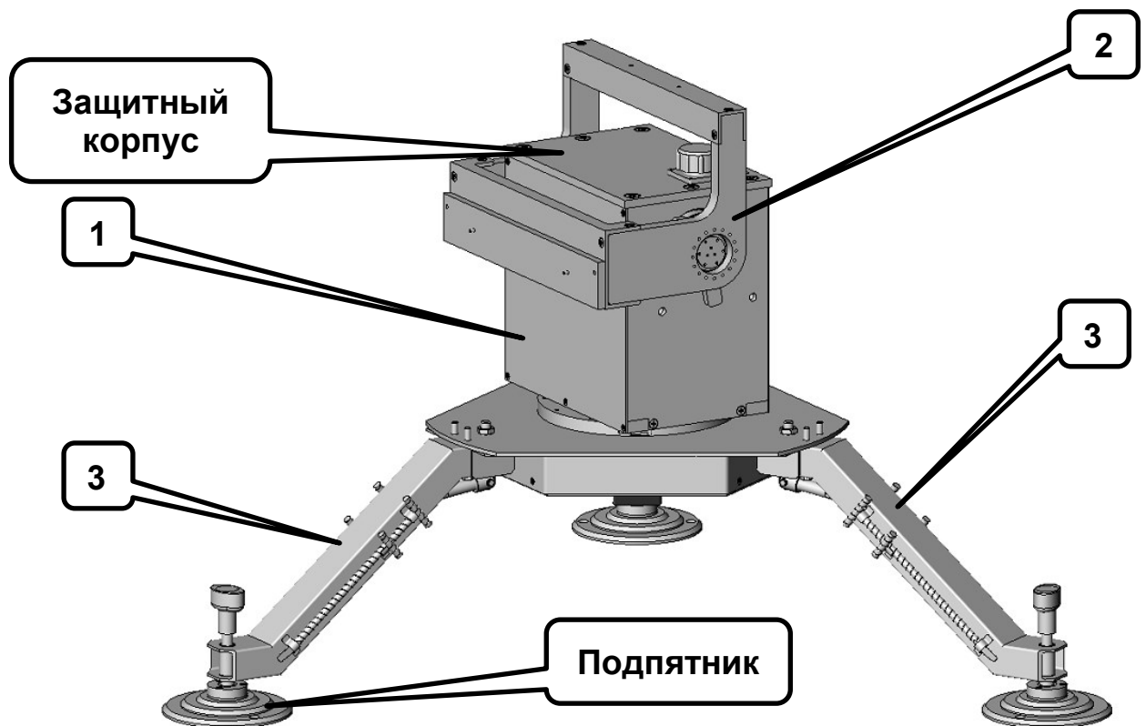
Рисунок 5 - Внешний вид ОПУ.
