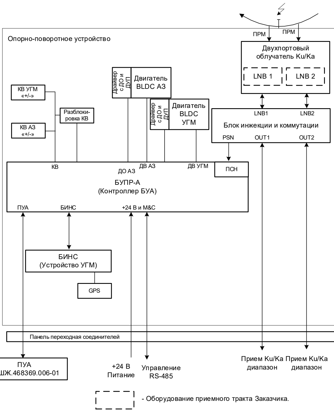
Рисунок 4 - Функциональная схема СССТ 1,2 м
