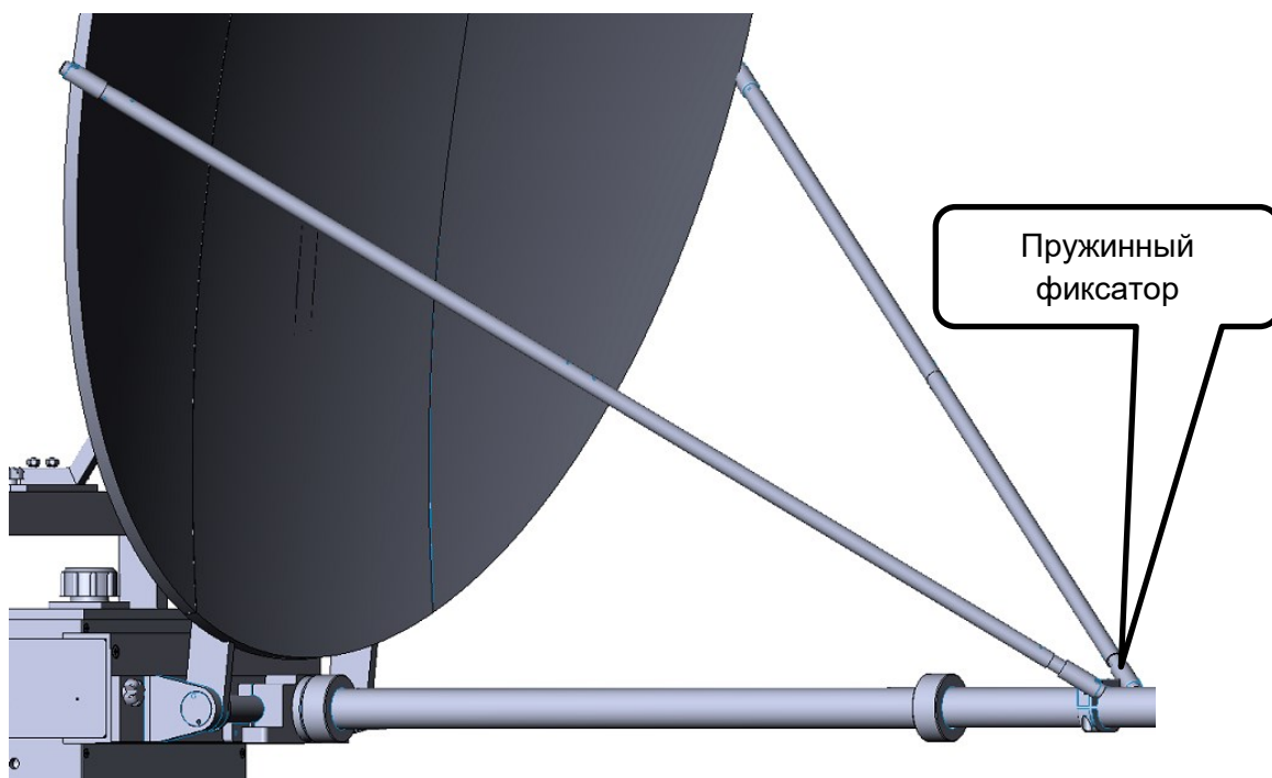
Рисунок 25 - Сборка и установка стоек держателя облучателя
