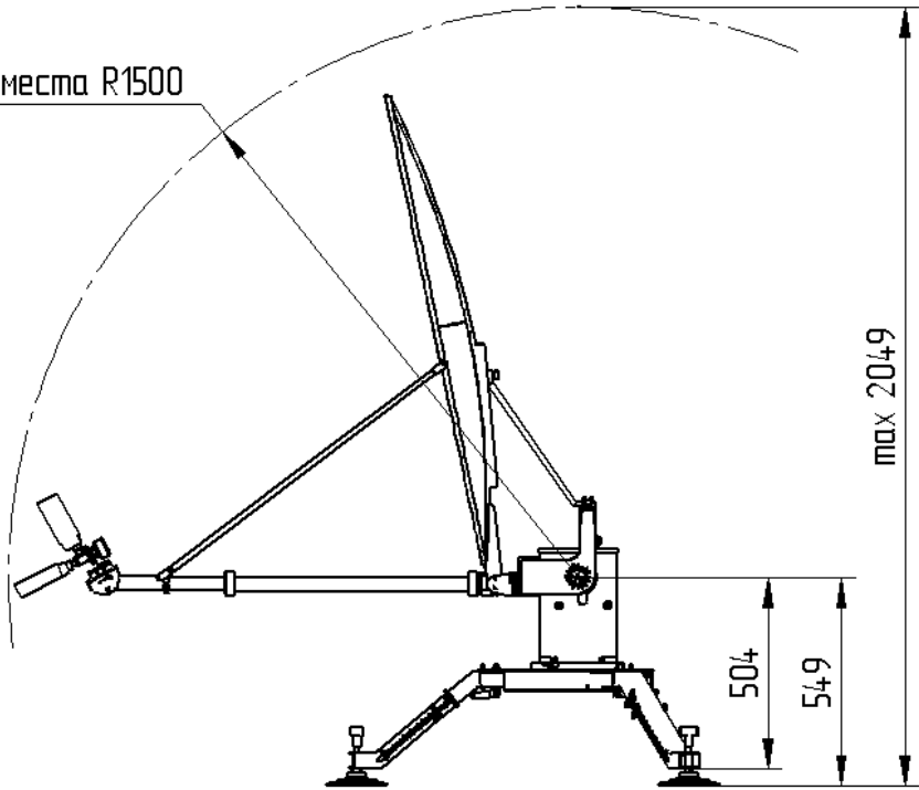
Рисунок 1 - Габаритный чертеж антенны в развернутом состоянии
