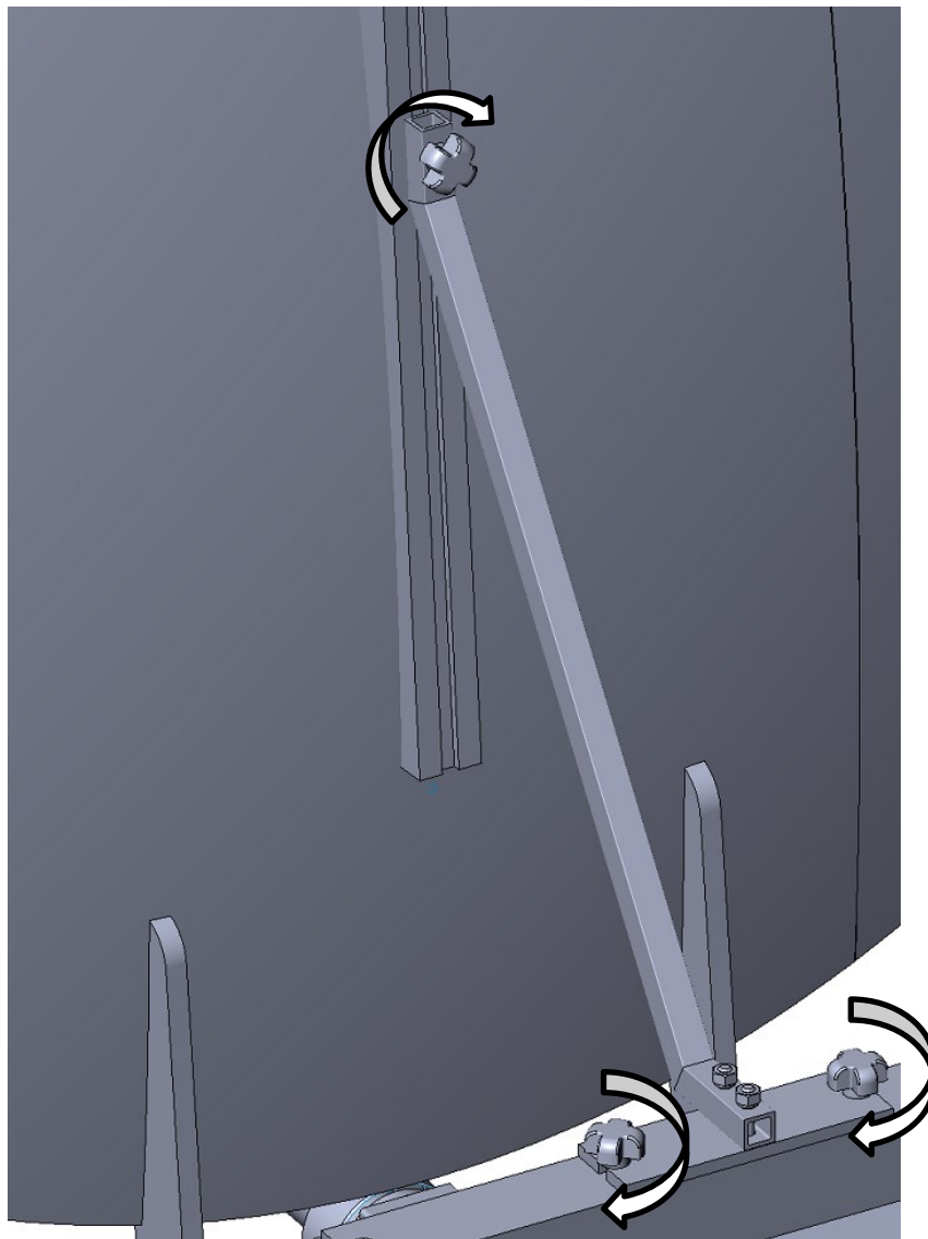
Рисунок 22 – Стыковка основного лепестка рефлектора (№1) с опорно-поворотным устройством
