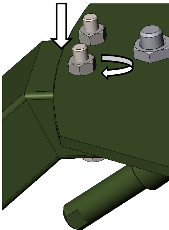
Рисунок 20 – Стыковка опорно-поворотной платформы на опорные лапы
