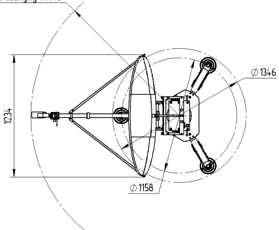
Рисунок 2 - Габаритный чертеж антенны в развернутом состоянии
