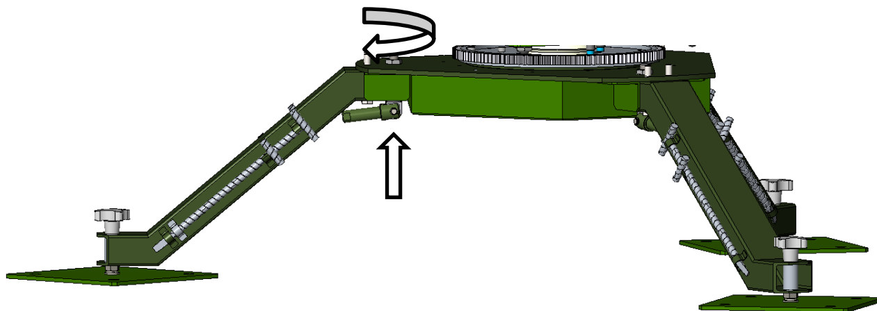
Рисунок 19 – Установка опорных лап
